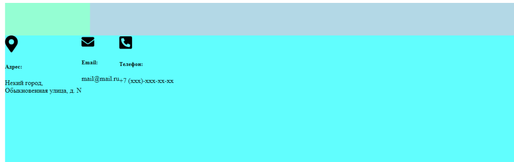
Рисунок 18 – Подвал flex-контейнер
