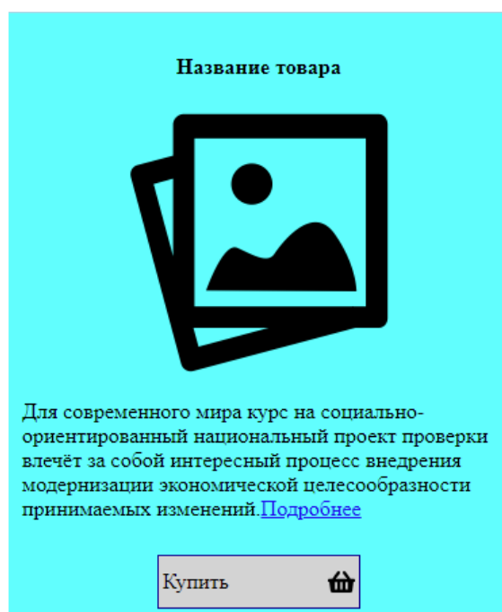
Рисунок 22 – Карточка товара
