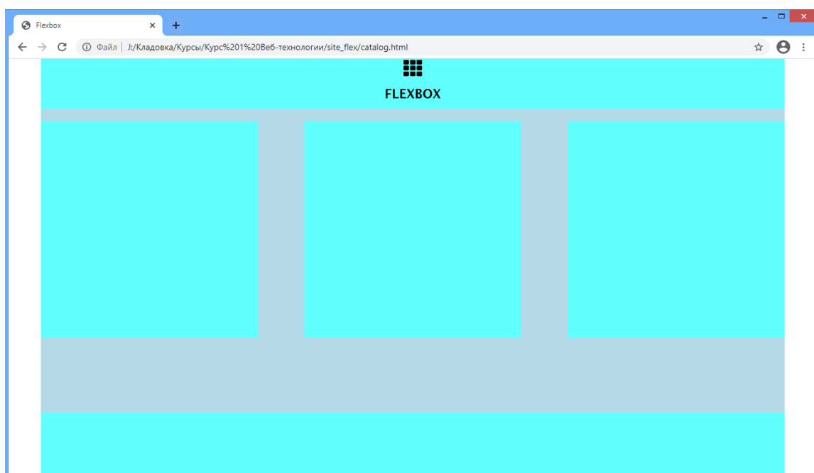
Рисунок 21 – Макет страницы
