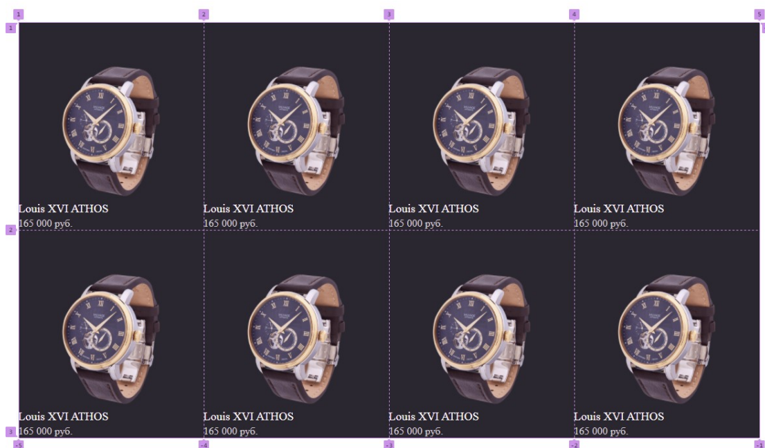
Рисунок 55 – Каталог
