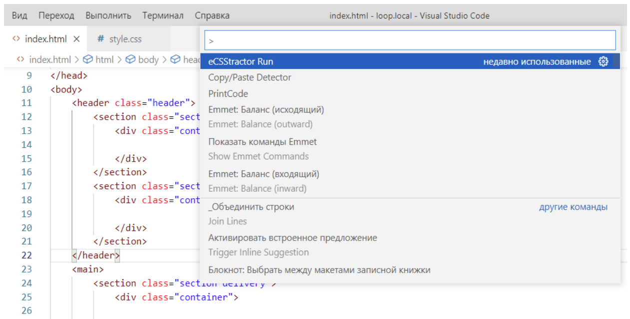
Рисунок 27 – Палитра команд
