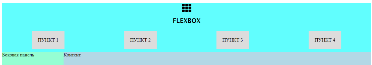
Рисунок 13 – Задание отступов
