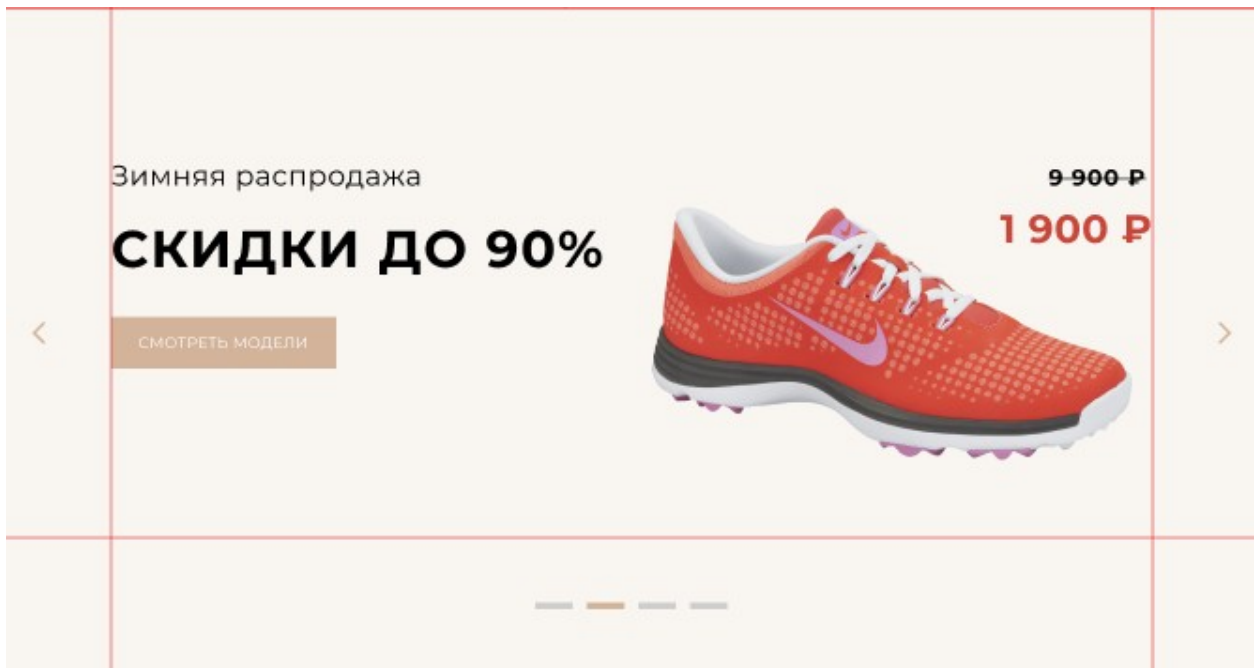
Рисунок 33 – Структура слайдера
