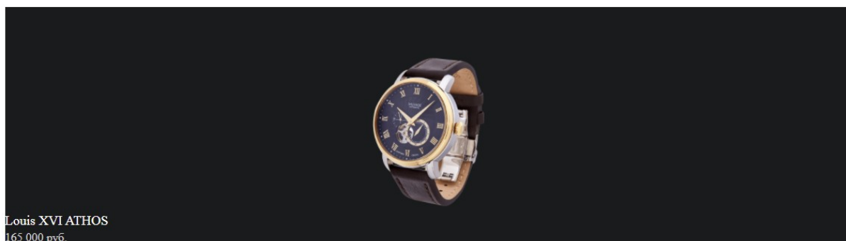
Рисунок 54 – Элемент каталога
