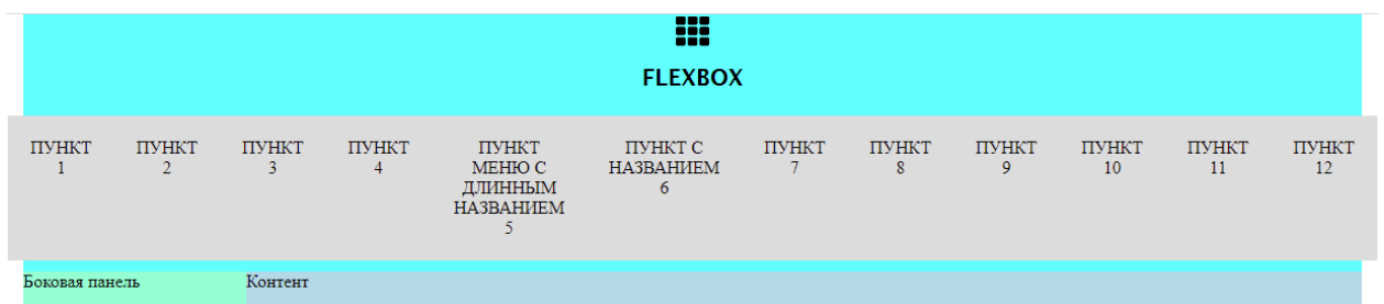
Рисунок 14 – Переполнение контейнера
