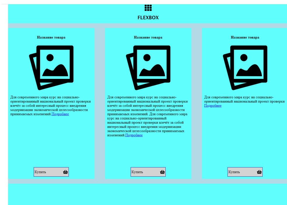
Рисунок 23 –Карточки товаров
