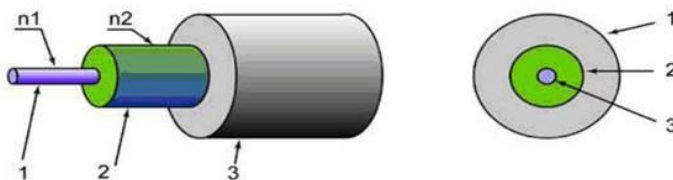
Рисунок 5. Структура оптоволоконного кабеля: 1 – сердцевина с показателем преломления n_1 ; 2 – отражающая оболочка с показателем преломления n_2 , n_1 > n_2 ; 3 – защитное покрытие.
