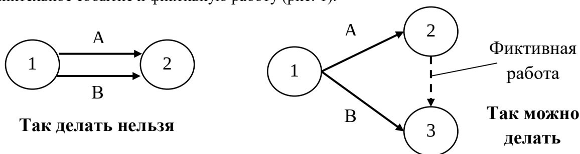
Рис. 1. Пример решения проблемы связей событий в сетевом графике
