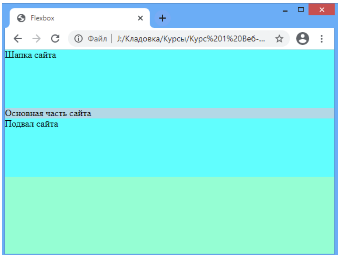
Рисунок 4 – Высота контейнера равна высоте окна браузера
