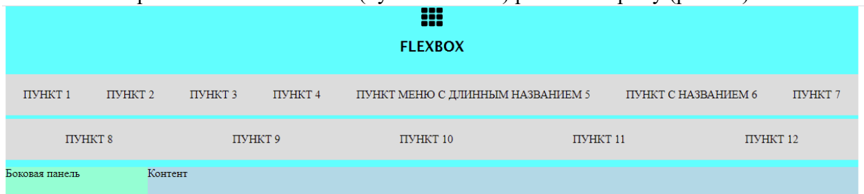
Рисунок 16 – Адаптация меню под всю ширину родителя
