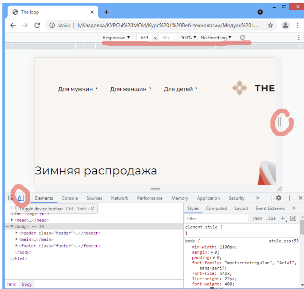
Рисунок 41 – Панель переключения устройств
