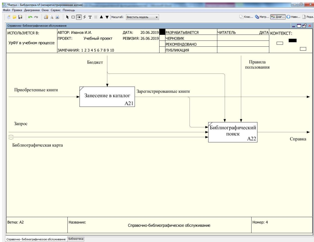
Рисунок 7.37 – Диаграмма декомпозиции блока «Справочно-библиографическое обслуживание»
