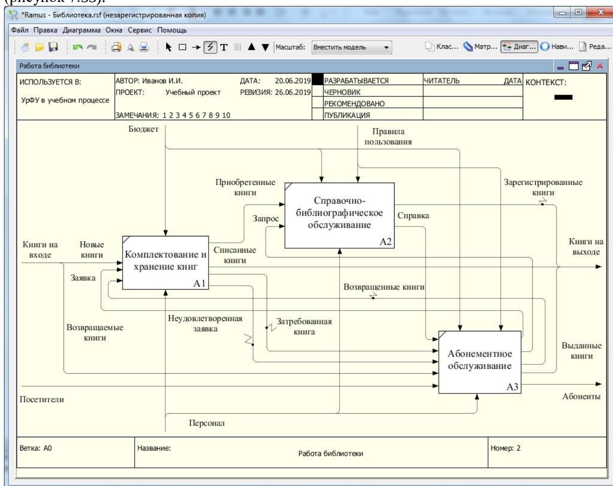
Рисунок 7.33. – Диаграмма декомпозиции контекстного блока «Работа библиотеки»
