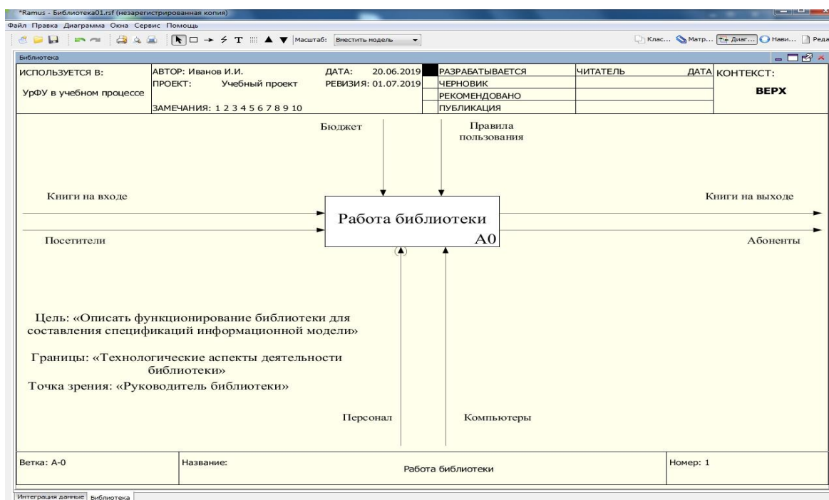
Рисунок 7.39 – Контекстная диаграмма модели TO-BE
