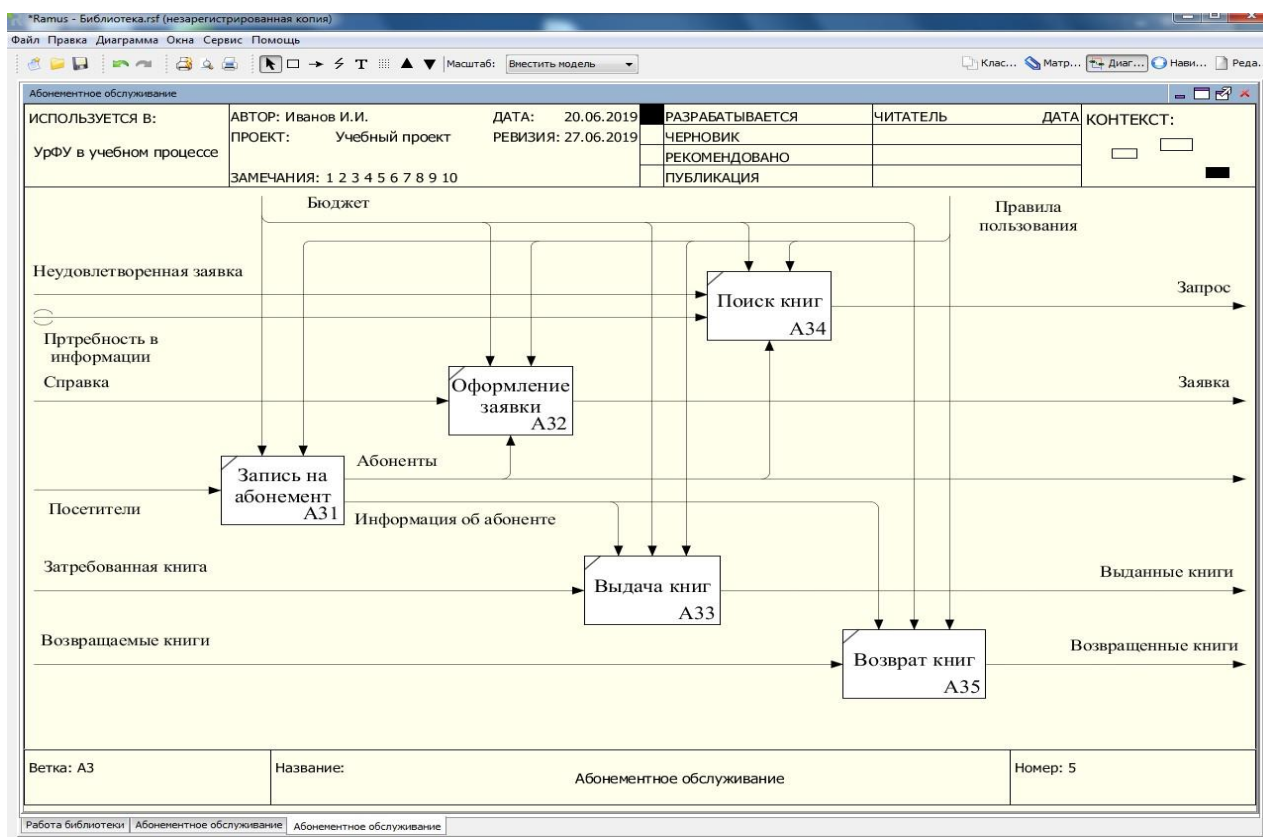
Рисунок 7.38 – Диаграмма декомпозиции блок «Абонементное обслуживание»
