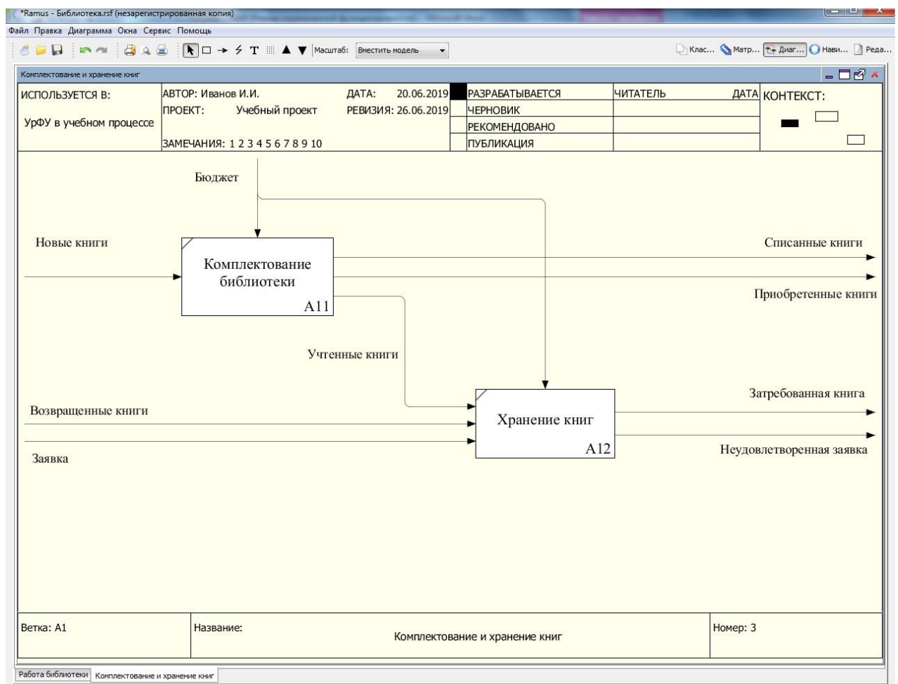
Рисунок 7.36 – Диаграмма декомпозиции блока «Комплектование и хранение книг»
