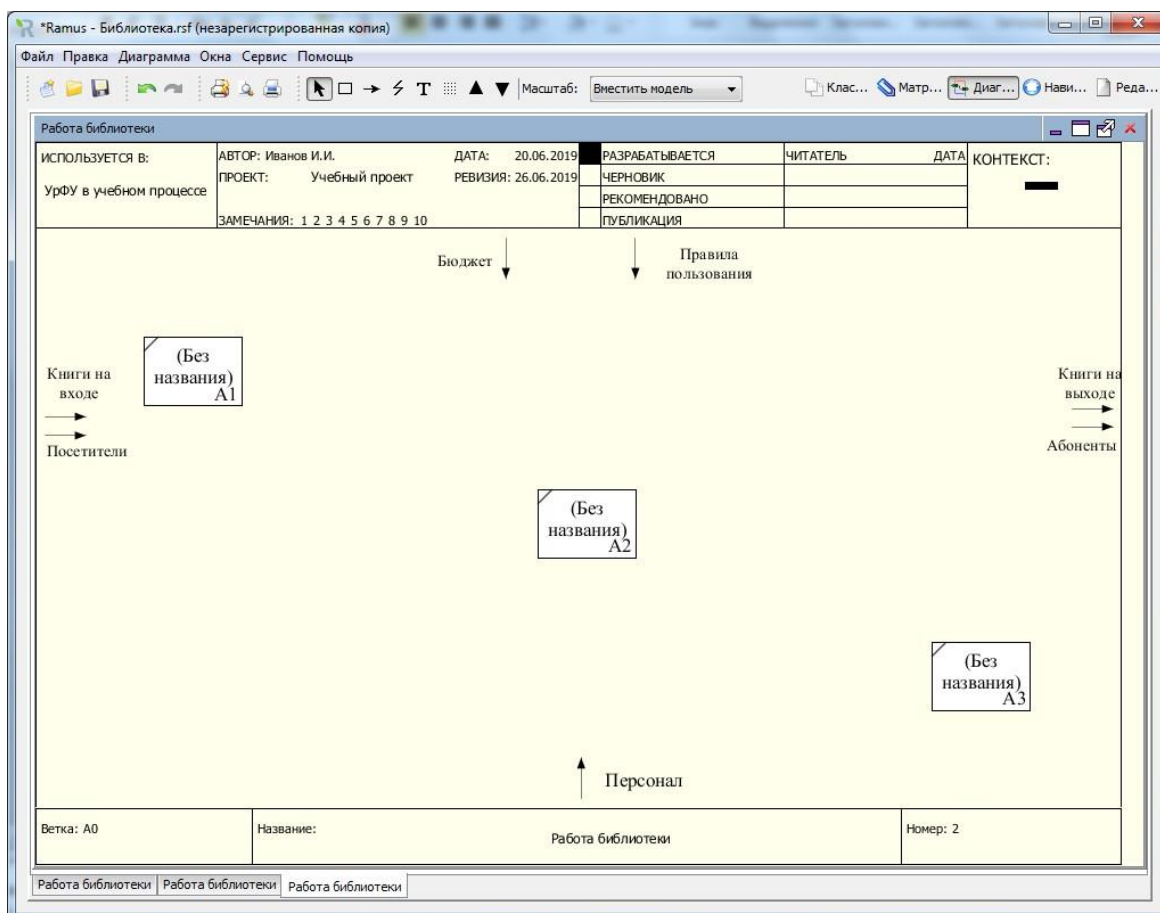
Рисунок 7.30 – Шаблон построения диаграммы декомпозиции
