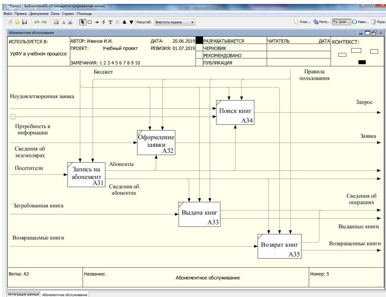
Рисунок 7.41 – Диаграмма декомпозиции блока «Абонементное обслуживание» модели TO-VE
