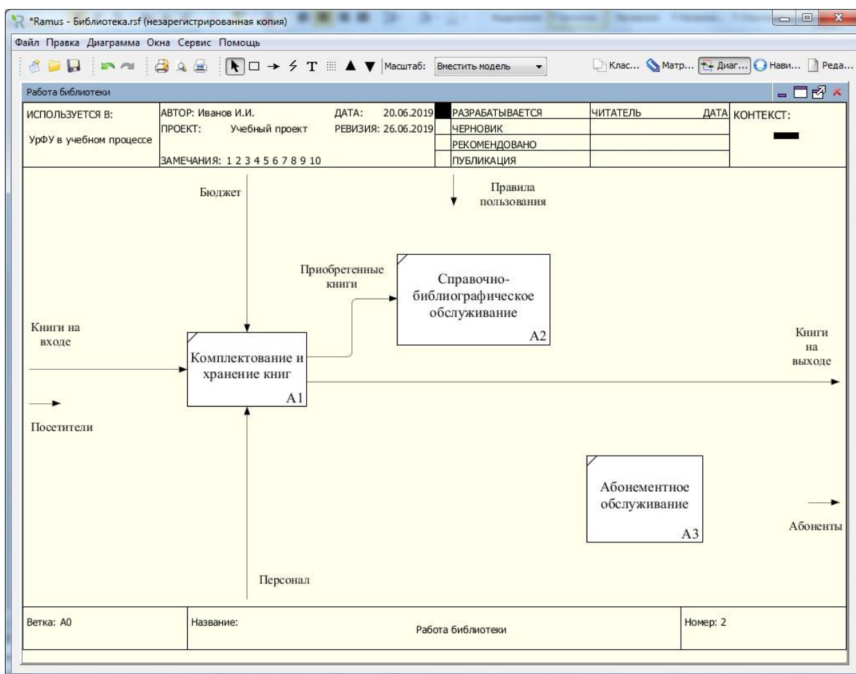
Рисунок 7.31 – Спецификация блока «Комплектование и хранение книг»
