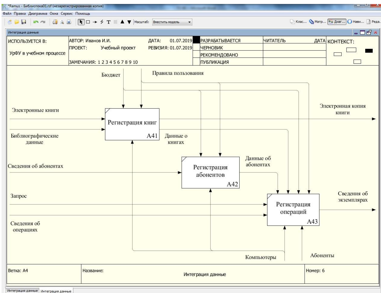
Рисунок 7.42 – Диаграмма декомпозиции блока «Интеграция данных» модели ТО-ВЕ
