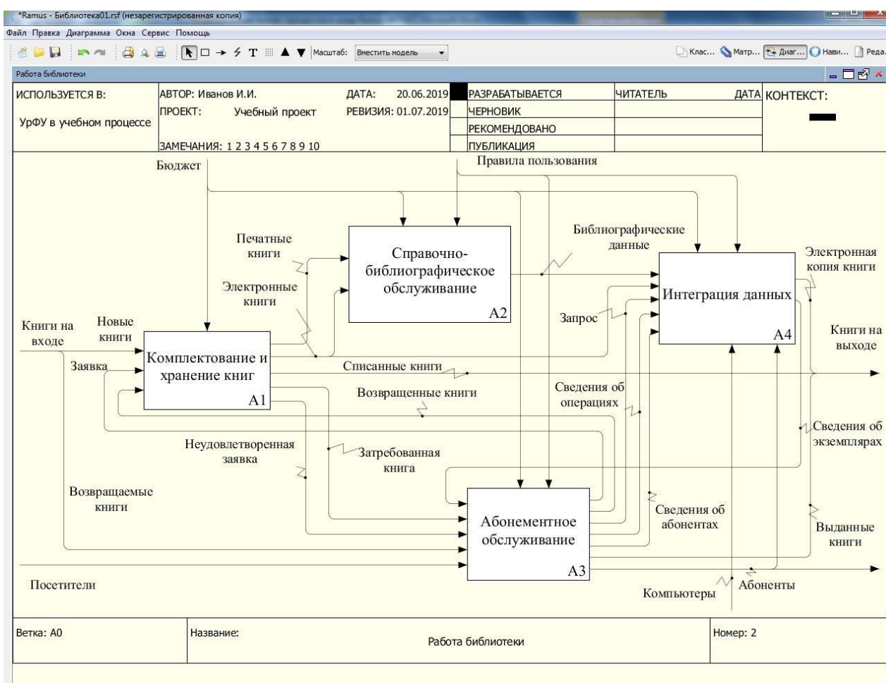
Рисунок 7.40 – Диаграмма декомпозиции контекстного блока модели TO-BE
