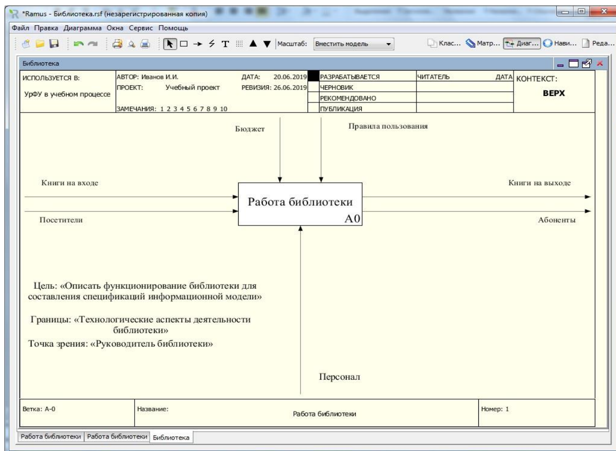
Рисунок 7.28 – Контекстная диаграмма
