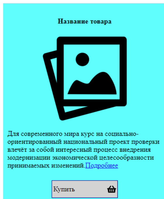
Рисунок 22 – Карточка товара
