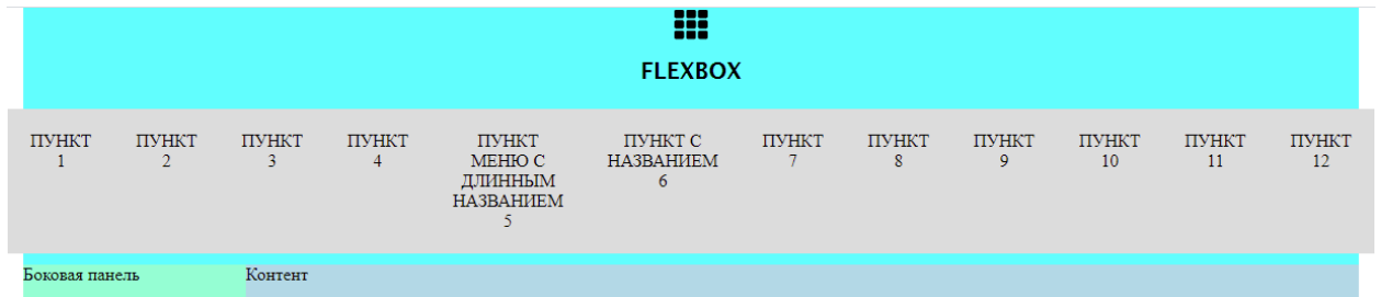
Рисунок 14 – Переполнение контейнера
