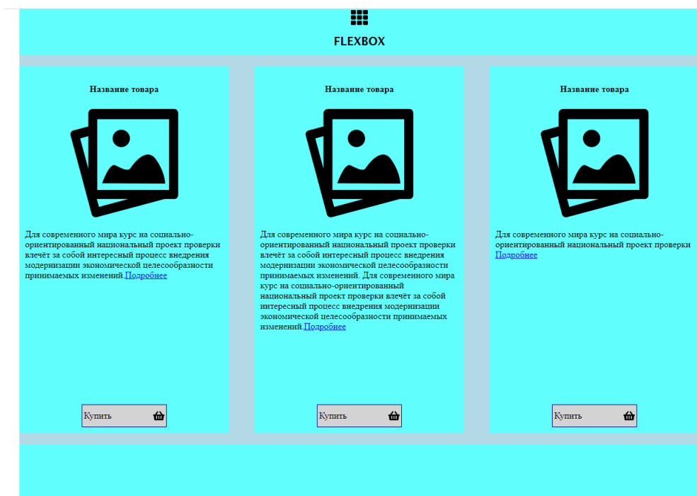
Рисунок 23 –Карточки товаров
