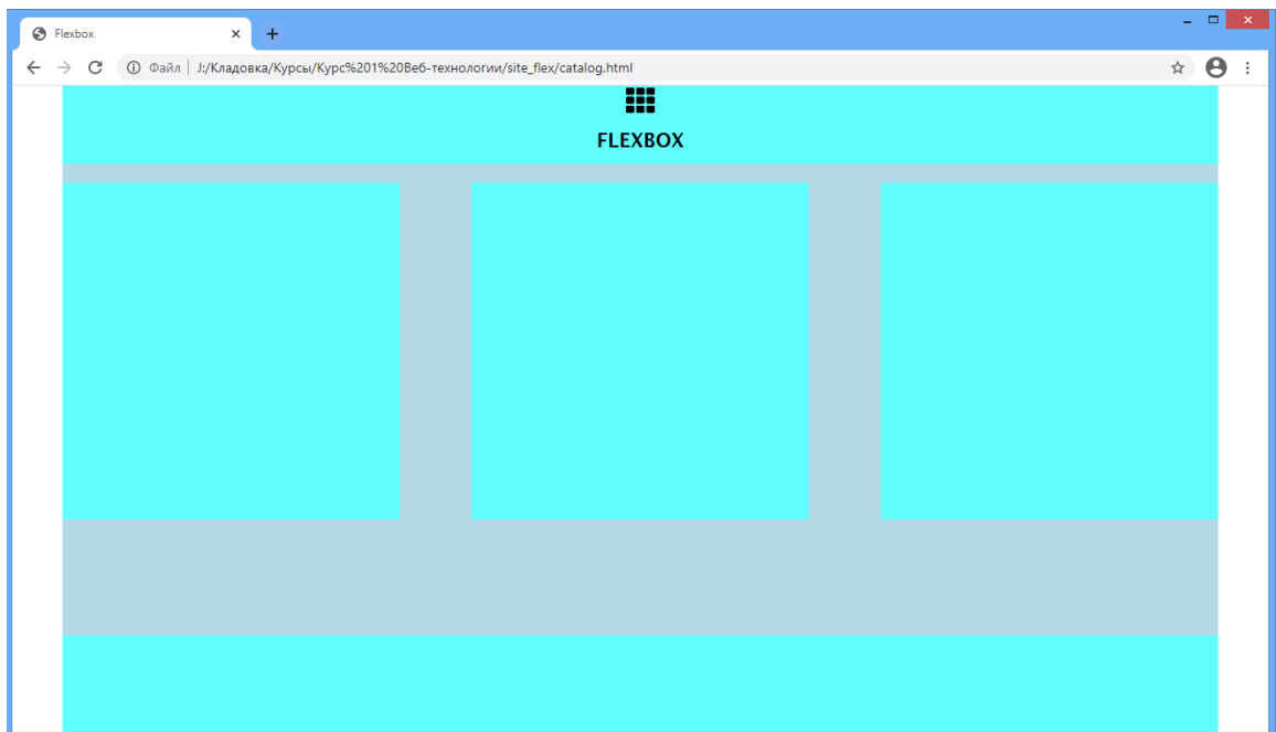
Рисунок 21 – Макет страницы
