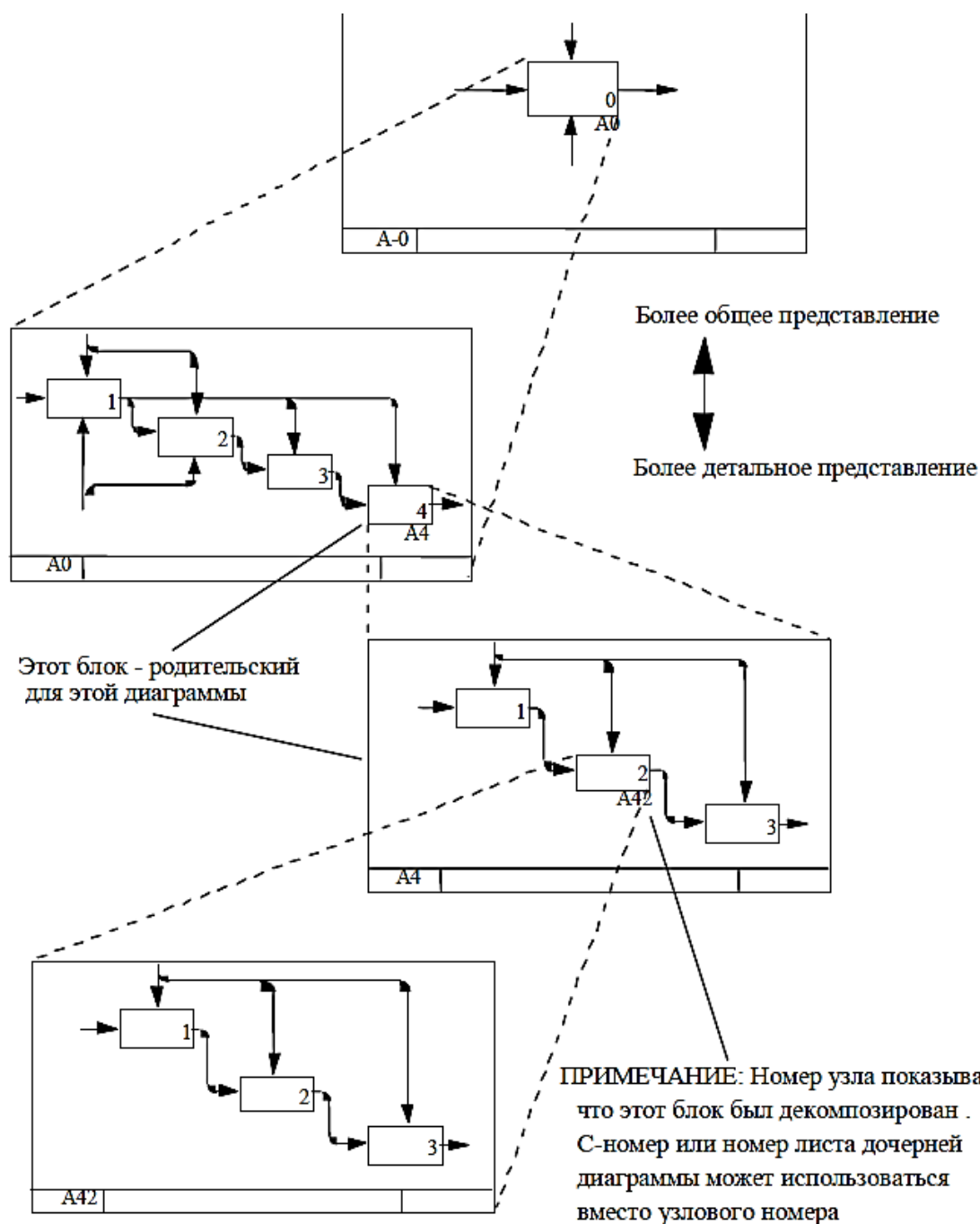
Рис. 4. Операция декомпозиции функциональных блоков в модели IDEF0
