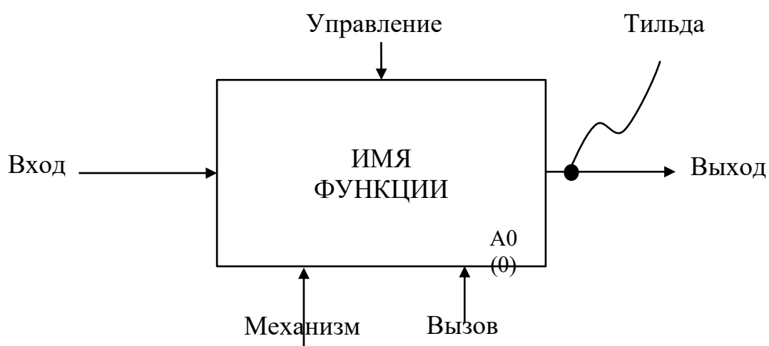
Рис. 3. Классическое представление функциональной модели IDEF0
