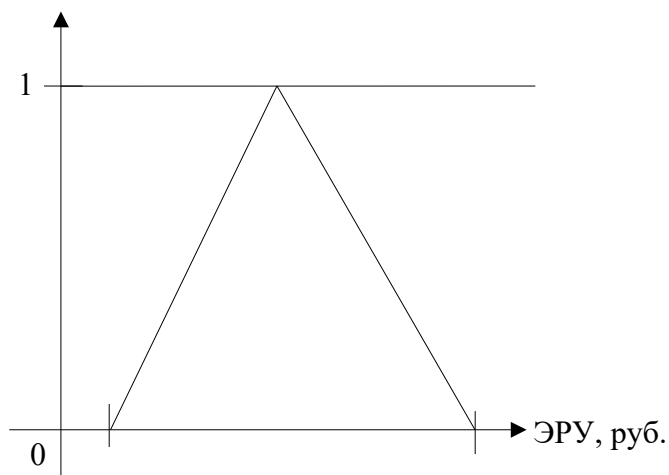
Рис. 2. Общий вид нечёткого треугольного числа экономического риска ущерба: \mathcal{E}РУ_{min}, \mathcal{E}РУ_{max} – минимальный и максимальный уровень возможного экономического риска ущерба; \mu(x) – функция принадлежности выражается через значение весового коэффициента k_i (формула 7)
