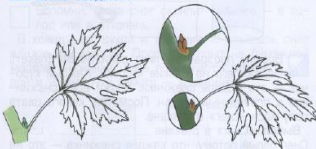
Лист летом
