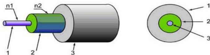
Рисунок 5. Структура оптоволоконного кабеля: 1 – сердцевина с показателем преломления n_1 ; 2 – отражающая оболочка с показателем преломления n_2 , n_1 > n_2 ; 3 – защитное покрытие.
