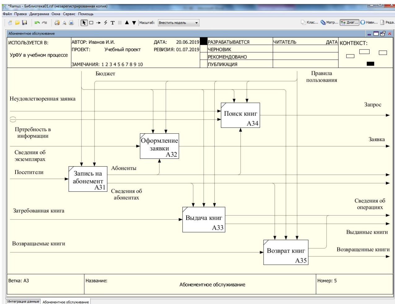
Рисунок 7.41 – Диаграмма декомпозиции блока «Абонементное обслуживание» модели TO-BE
