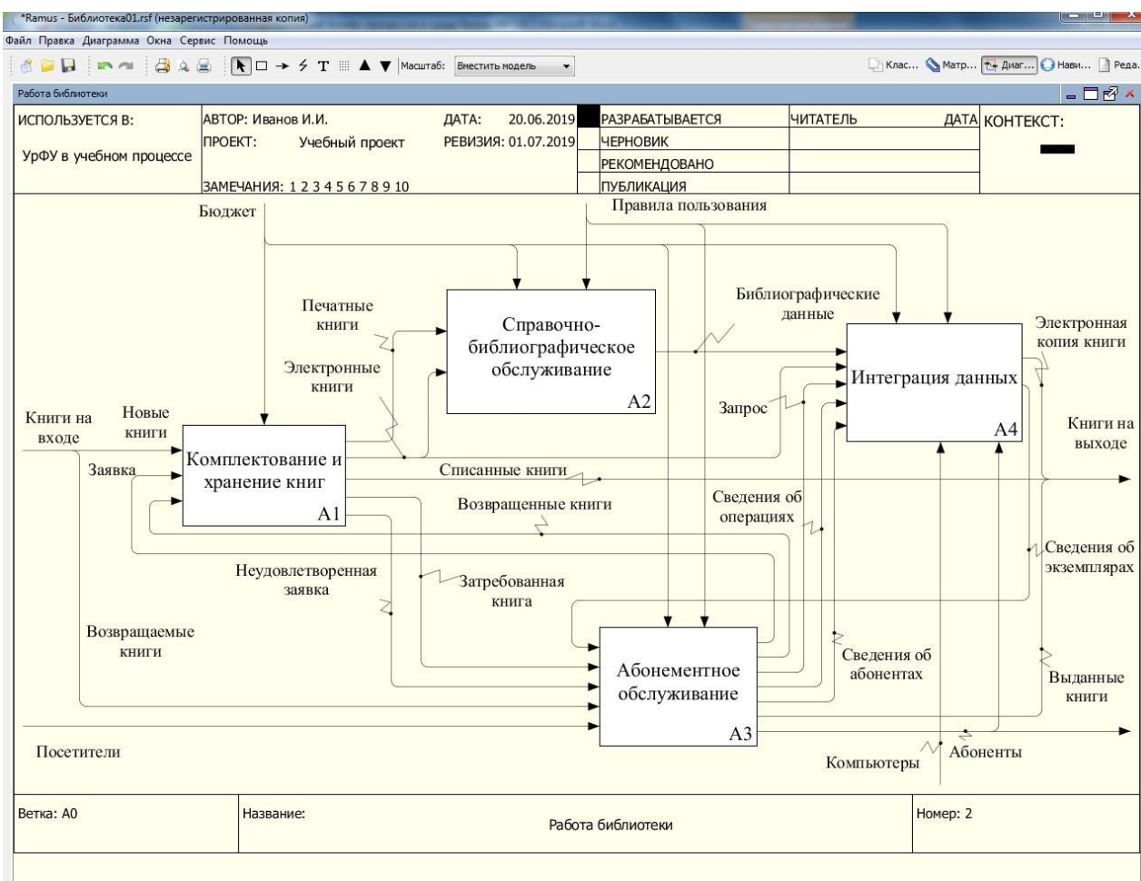
Рисунок 7.40 – Диаграмма декомпозиции контекстного блока модели TO-BE
