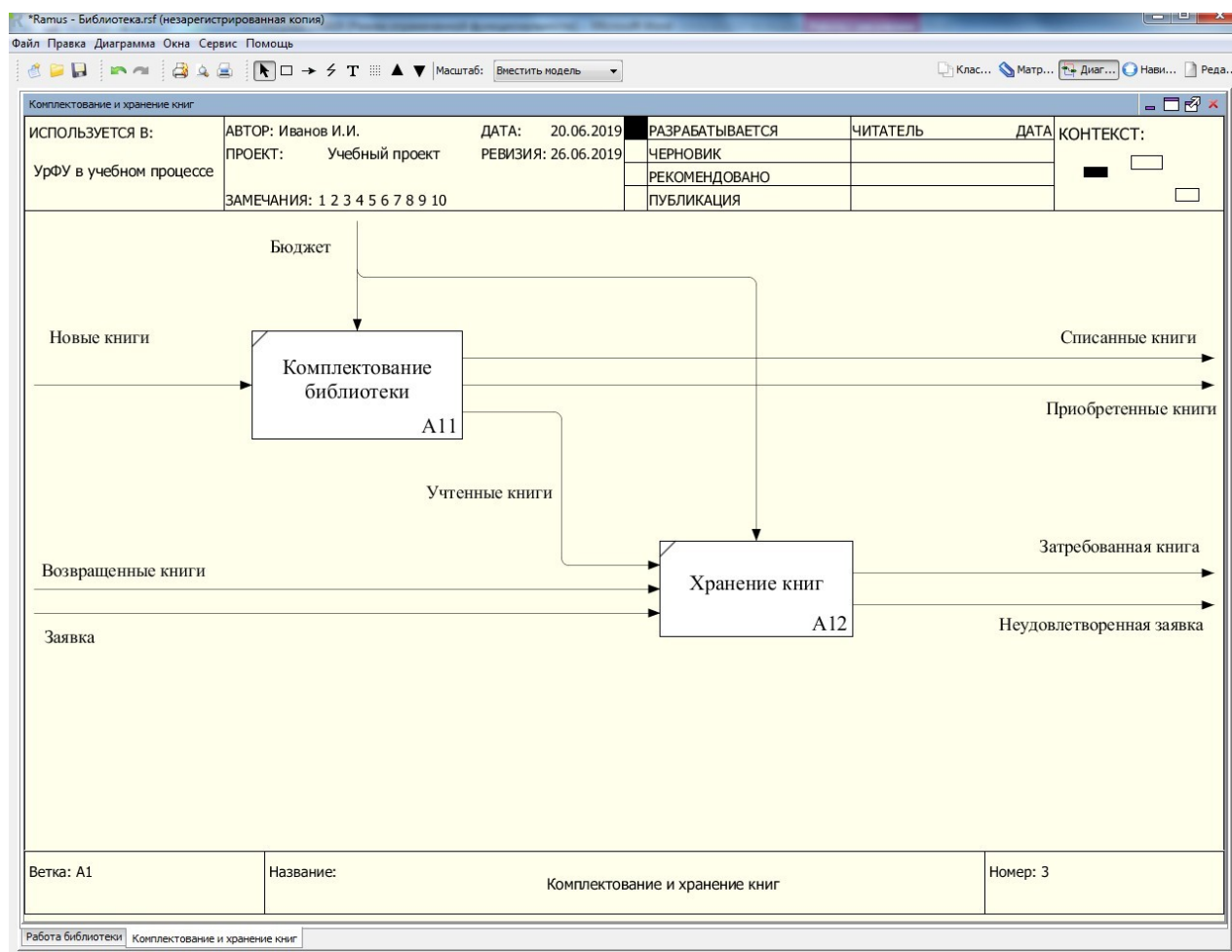
Рисунок 7.36 – Диаграмма декомпозиции блока «Комплектование и хранение книг»
