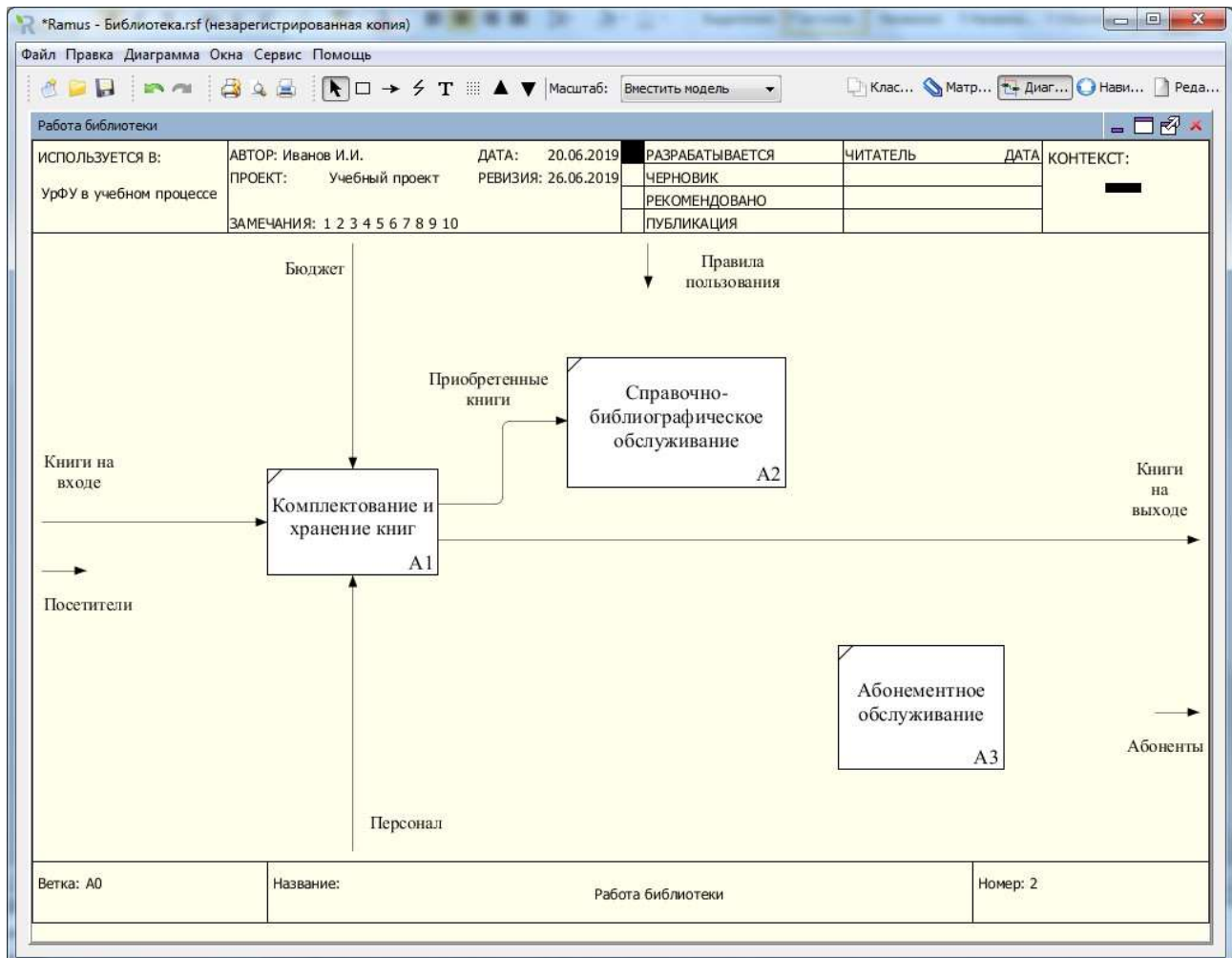
Рисунок 7.32 – Спецификация блока «Комплектование и хранение книг»
