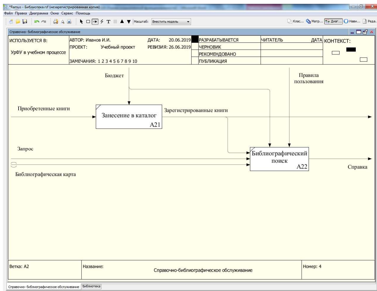
Рисунок 7.38 – Диаграмма декомпозиции блока «Справочно-библиографическое обслуживание»
