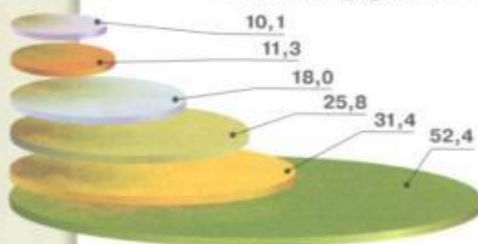
Площадь природных зон суши Земли (млн км 2 )
