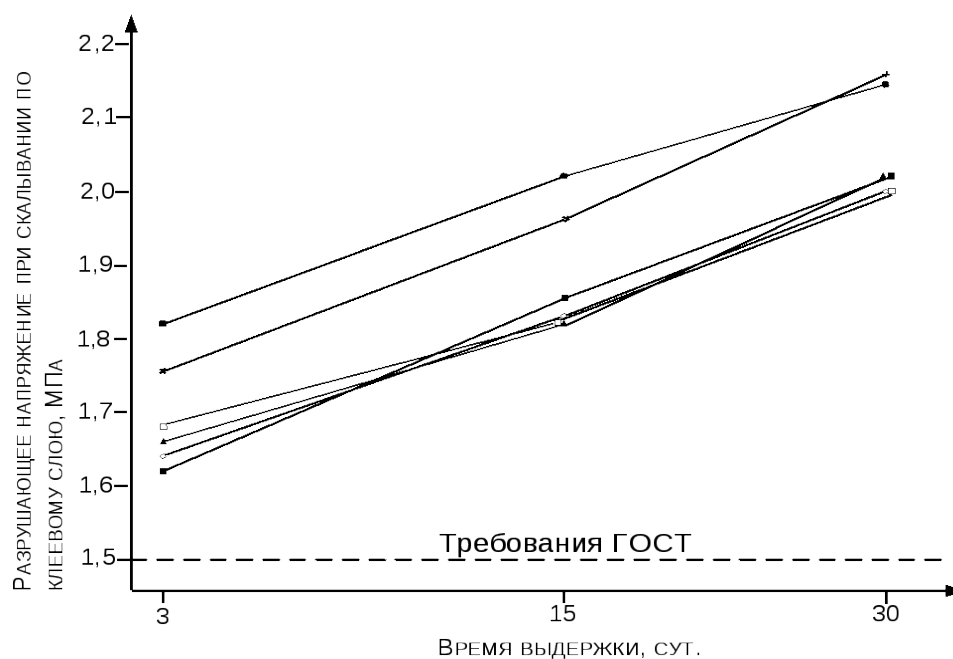
Рисунок 1 - Динамика разрушающего напряжения при скалывании по клеевому слою исследуемых образцов фанеры, T = 20 \pm 2^\circ\text{C} ; t = 3 - 30 суток, где ● – контрольный образец; ○ – образец 1; ▲ – образец 2; ■ – образец 3; □ – образец 4; х – образец 5
