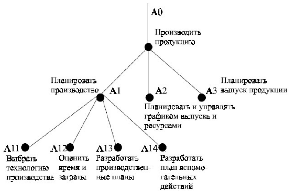
Рис. 1. Пример дерева узлов по методологии IDEF0
