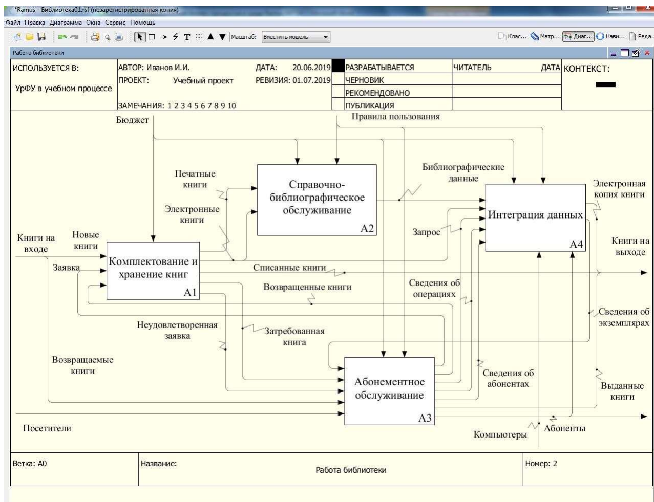
Рисунок 7.41 – Диаграмма декомпозиции контекстного блока модели ТО-ВЕ
