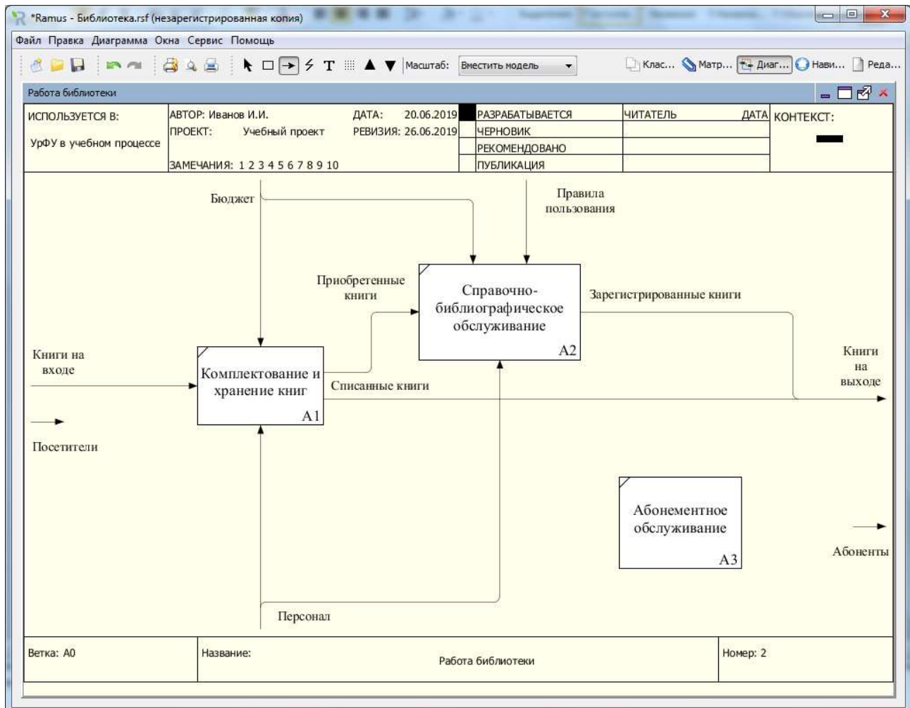
Рисунок 7.33 – Спецификация блока «Справочно-библиографическое обслуживание»
