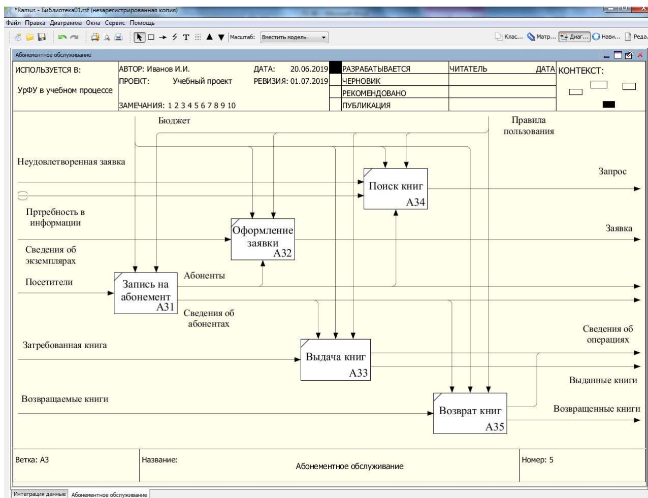
Рисунок 7.42 – Диаграмма декомпозиции блока «Абонементное обслуживание» модели ТО-ВЕ
