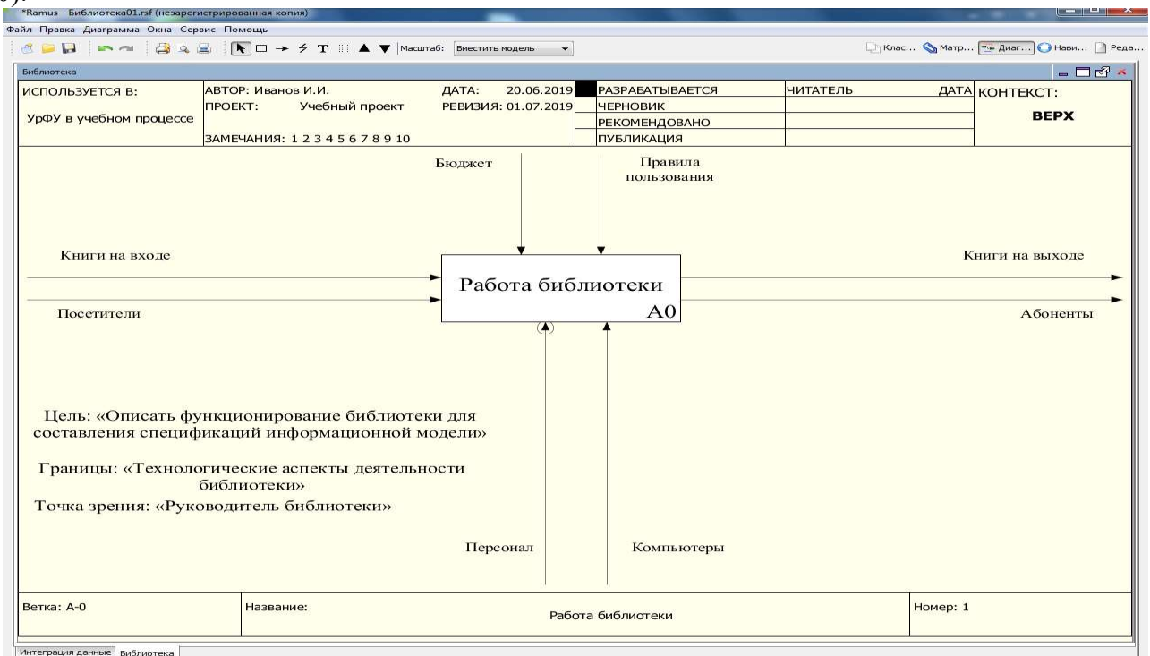
Рисунок 7.40 – Контекстная диаграмма модели ТО-ВЕ
