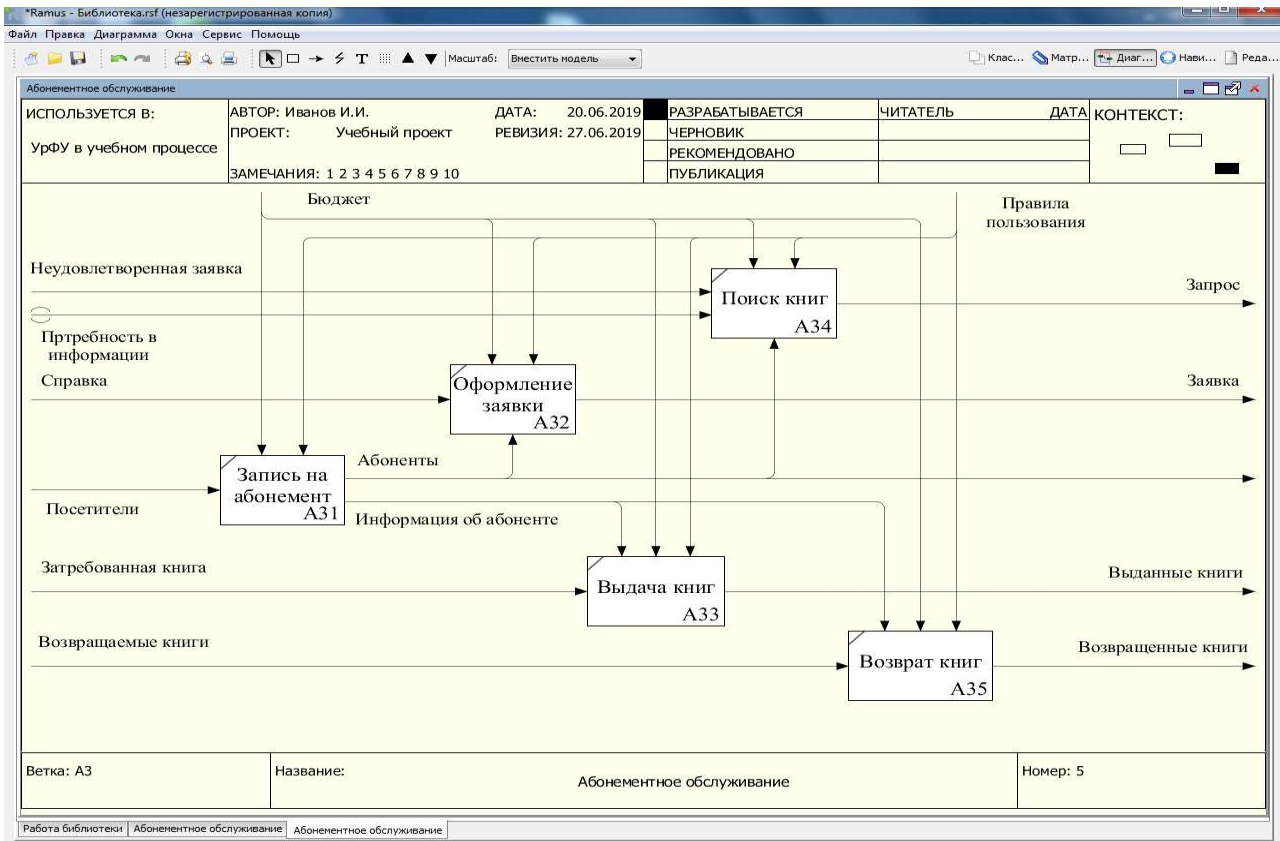
Рисунок 7.39 – Диаграмма декомпозиции блок «Абонементное обслуживание»
