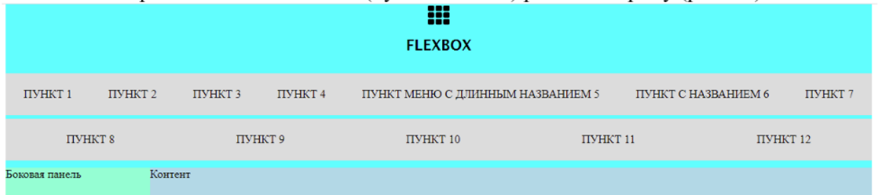
Рисунок 16 – Адаптация меню под всю ширину родителя
