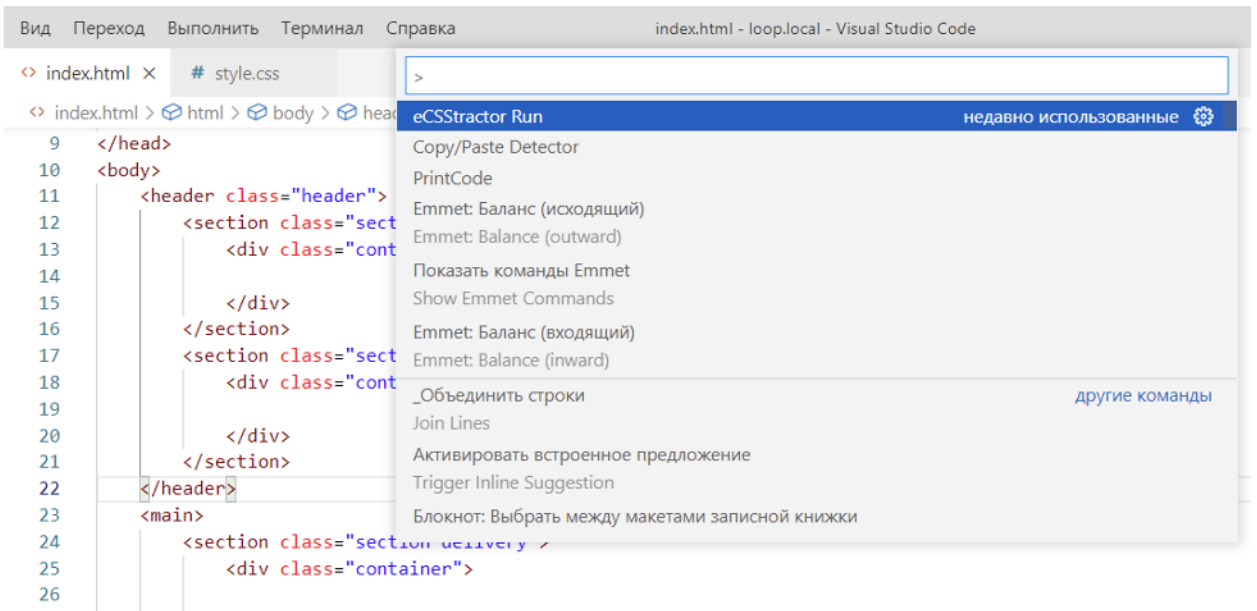
Рисунок 27 – Палитра команд
