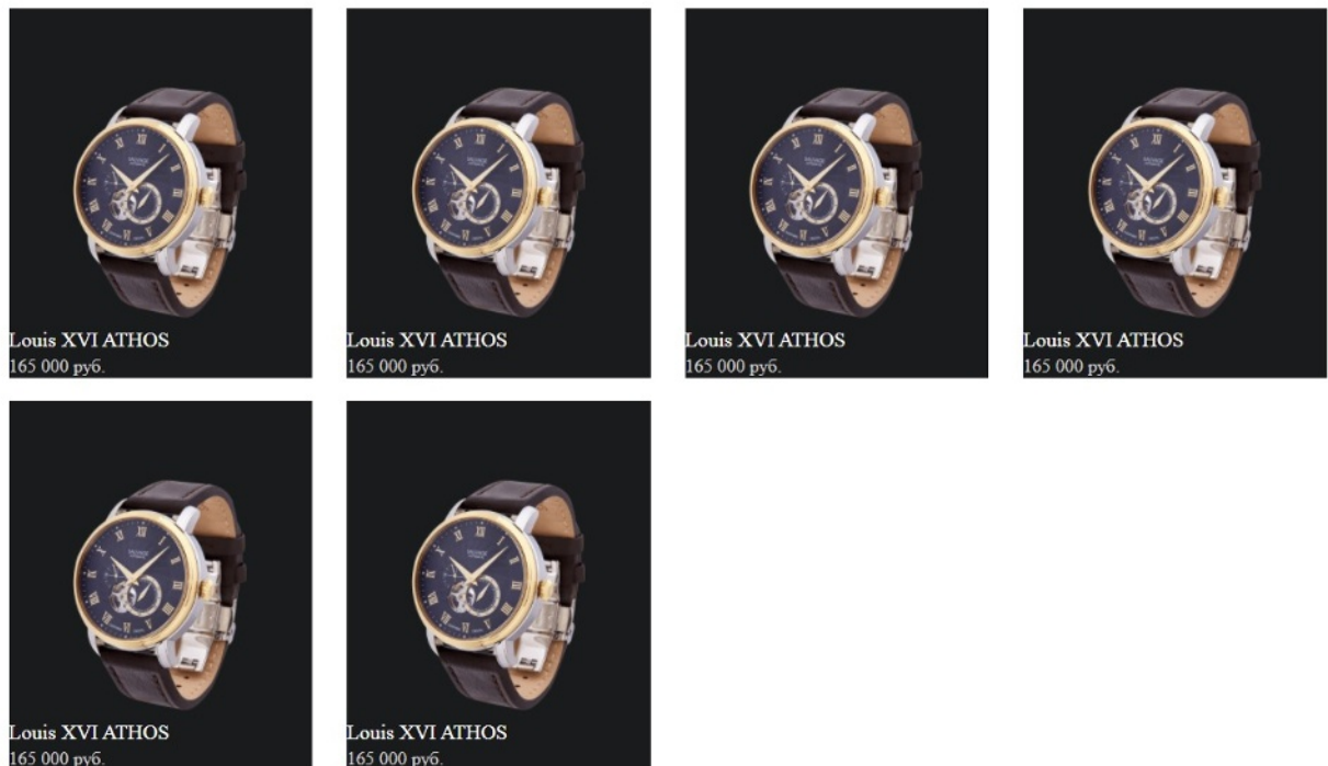
Рисунок 57 – Структура сетки
