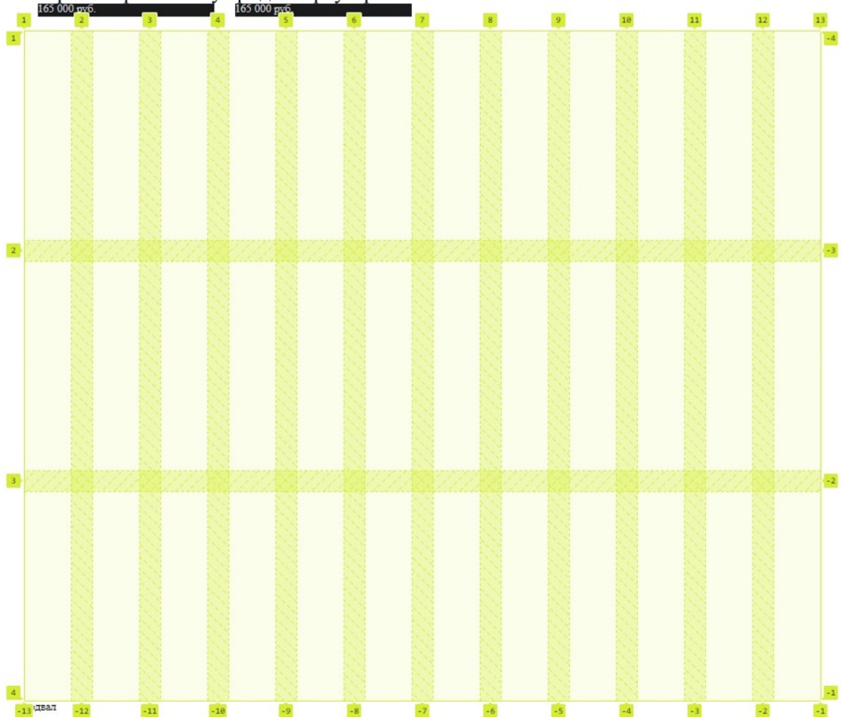
Рисунок 62 – Грид-сетка
