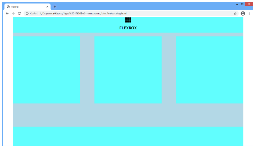
Рисунок 21 – Макет страницы
