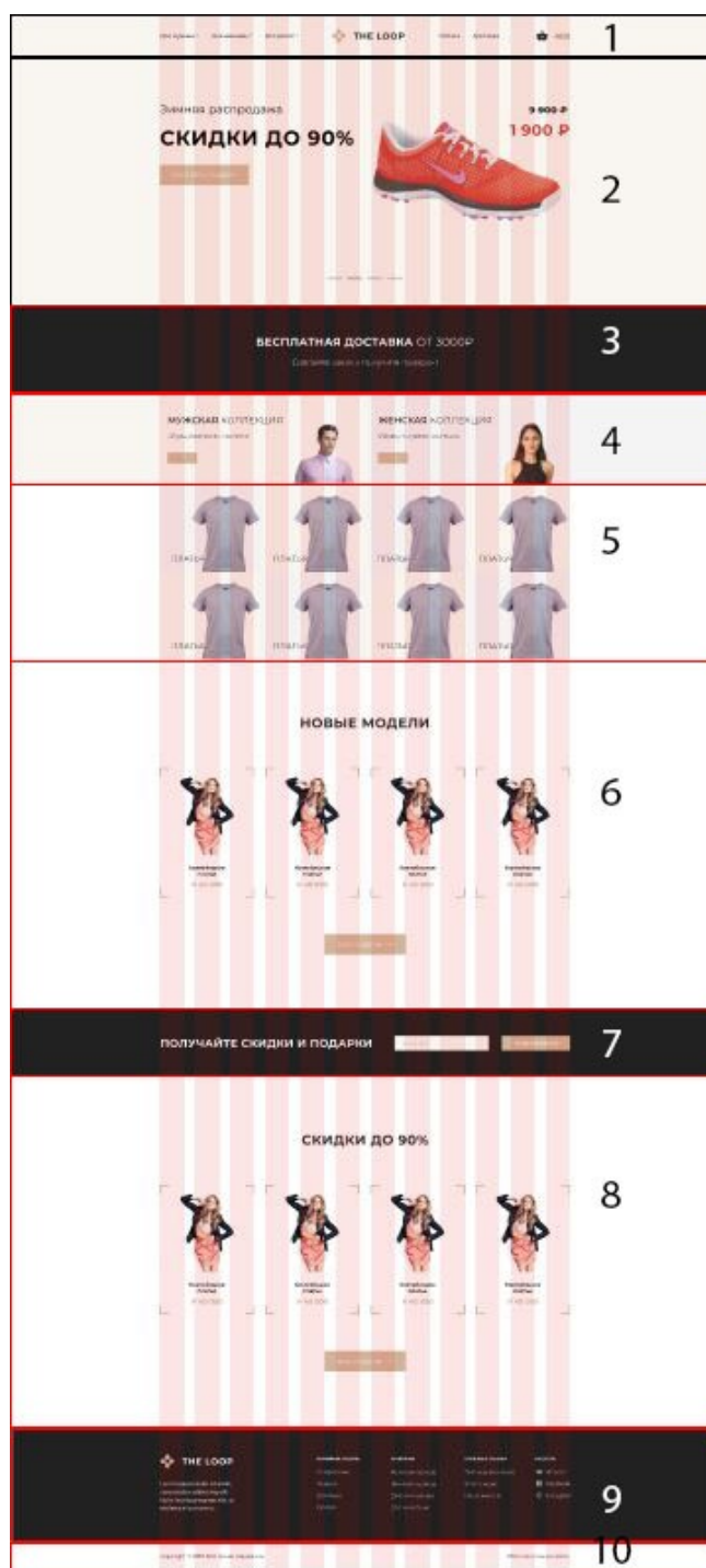
Рисунок 26 – Разделы сайта
