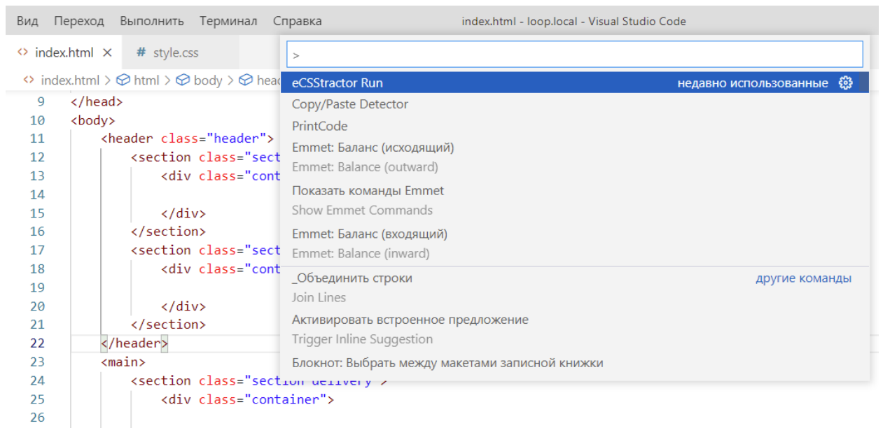
Рисунок 27 – Палитра команд
