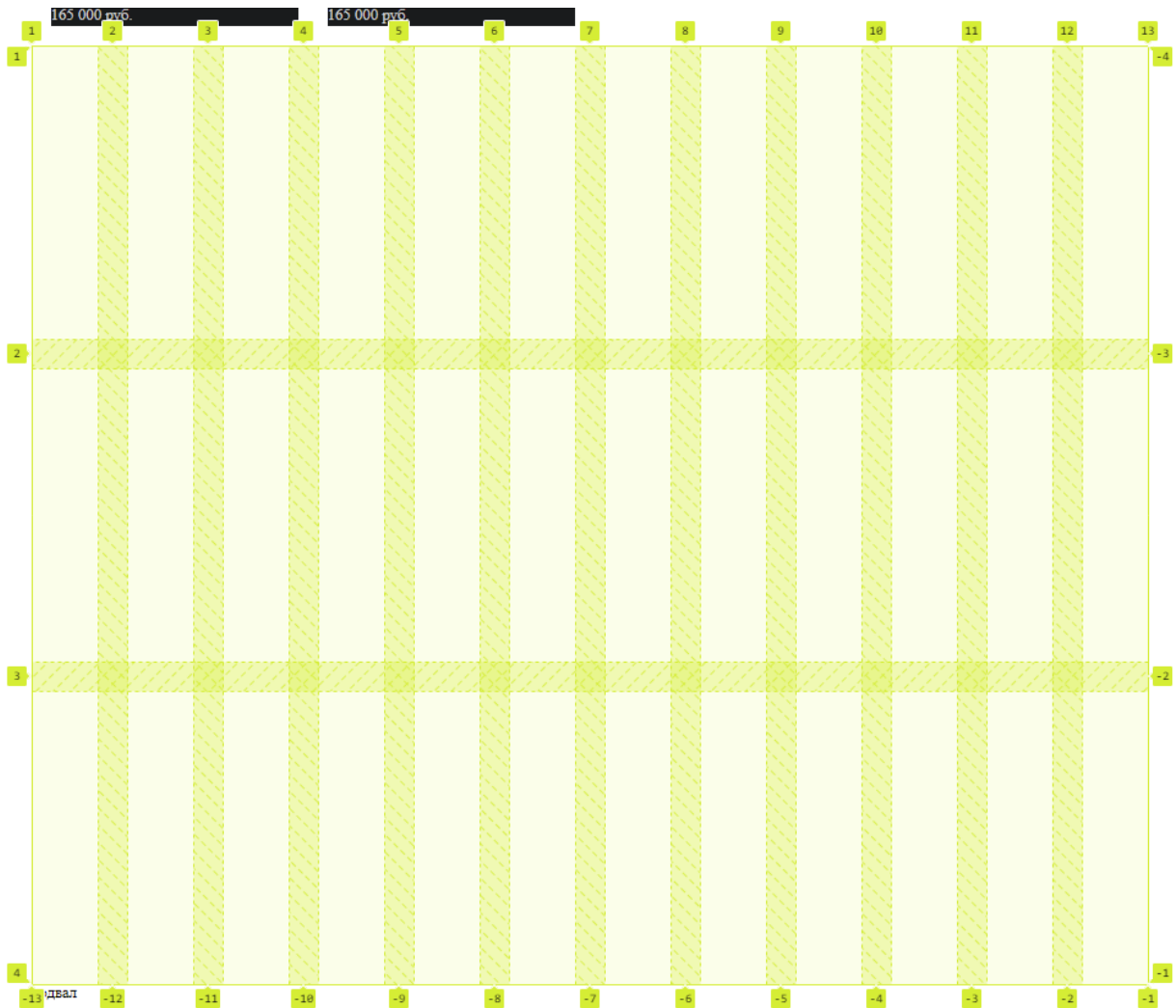
Рисунок 13 – Грид-сетка
