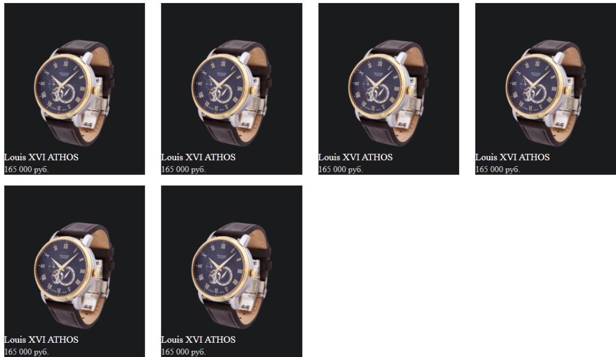
Рисунок 8 – Структура сетки
