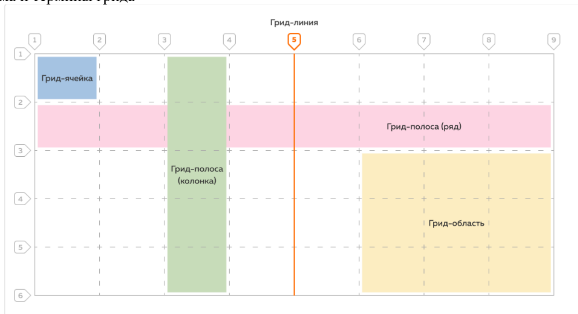
Рисунок 1 – Грид-сетка
