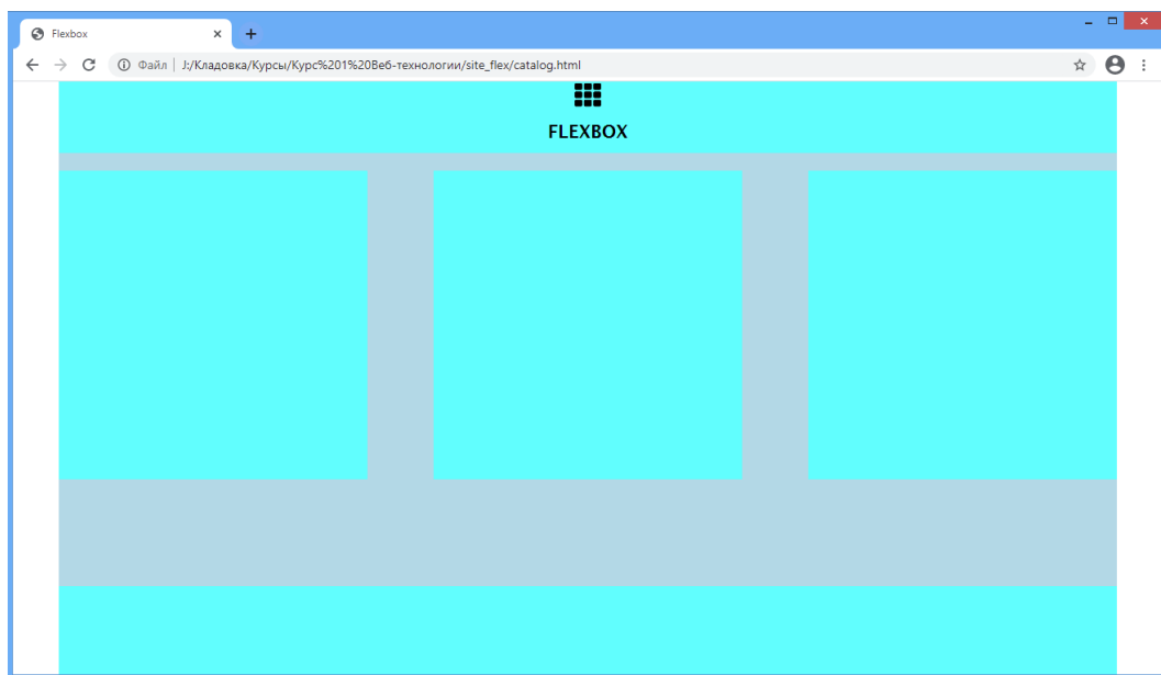
Рисунок 21 – Макет страницы
