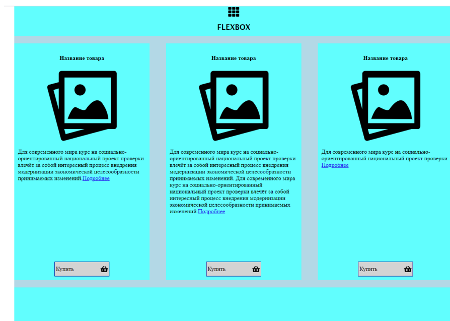
Рисунок 23 –Карточки товаров
