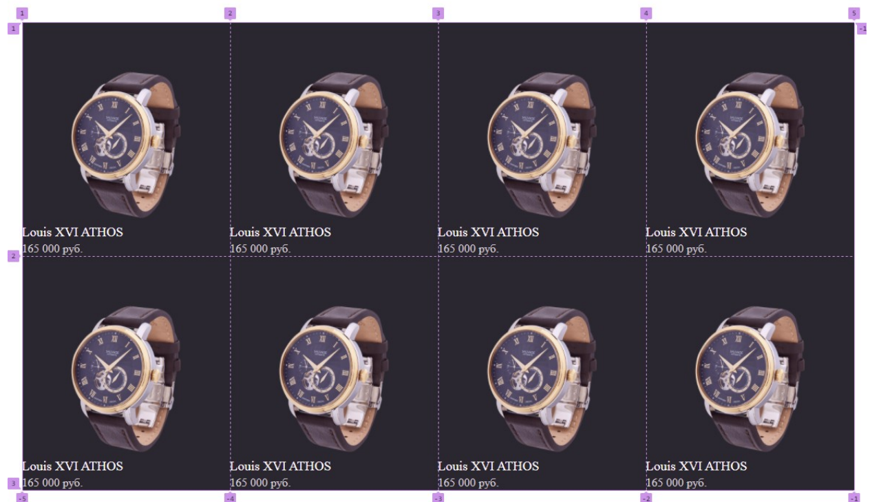
Рисунок 55 – Каталог
