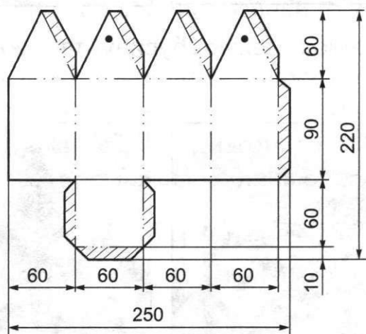
Чертёж развёртки фонарика
