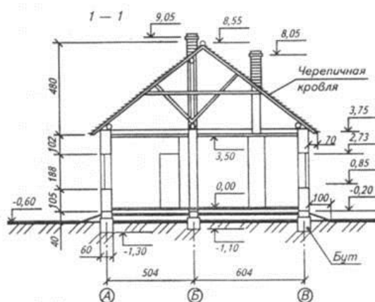
Рис. 8. Сельская библиотека: разрез
