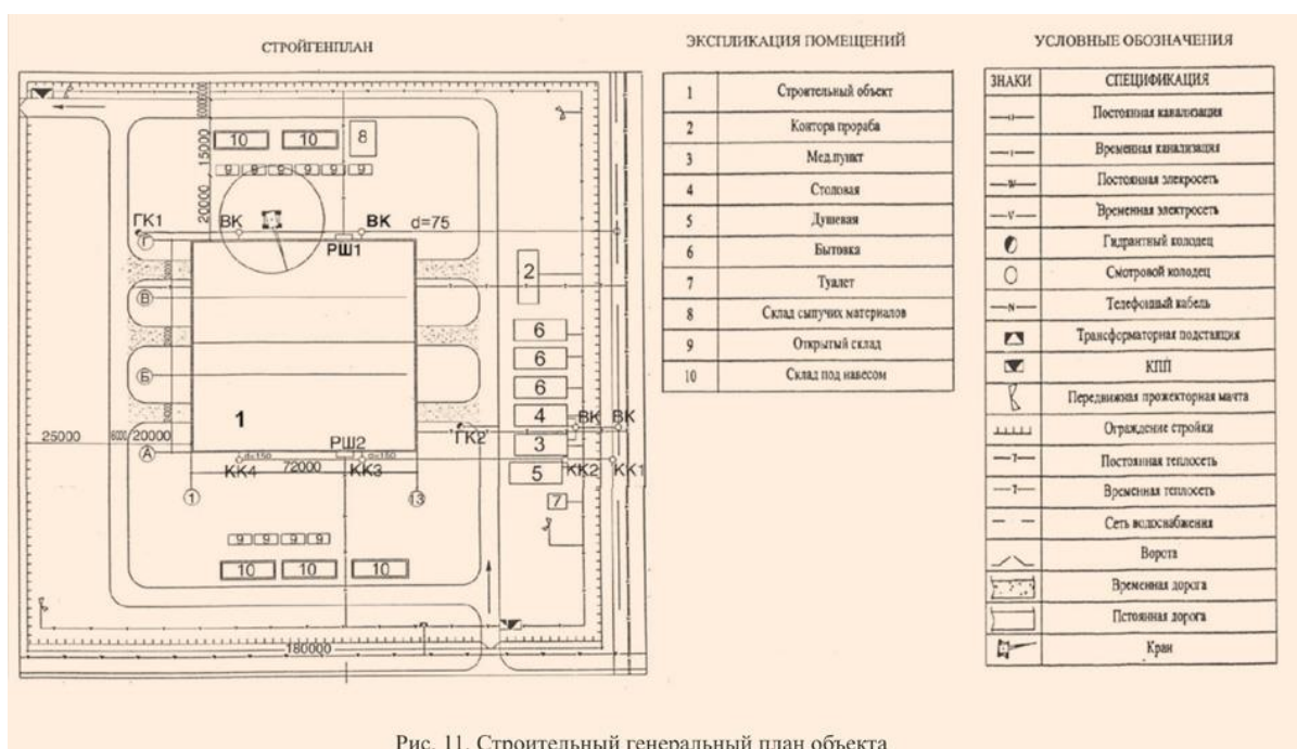
Рис. 11. Строительный генеральный план объекта
