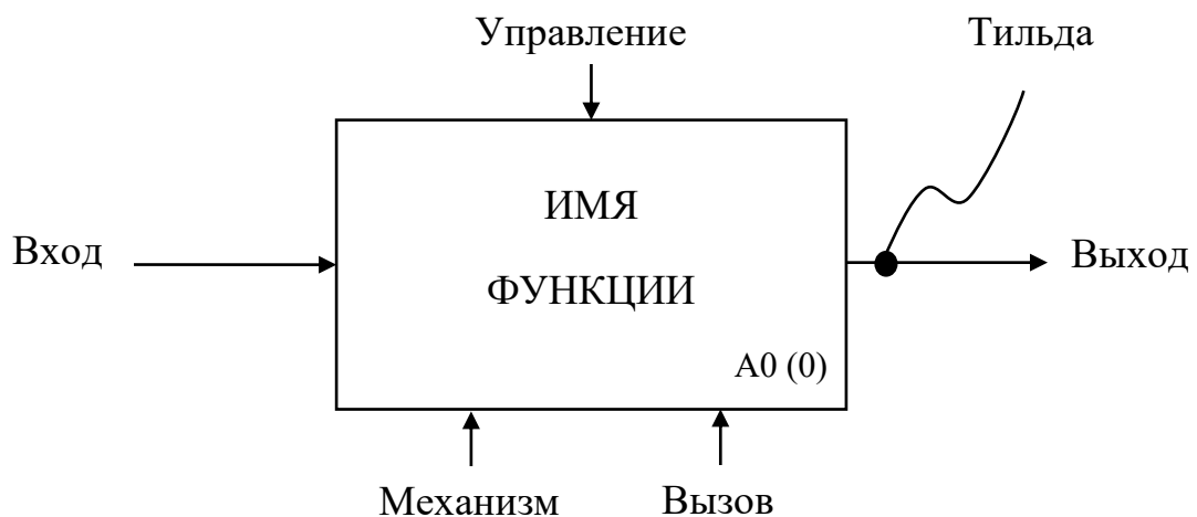
Рис. 3. Классическое представление функциональной модели IDEF0
