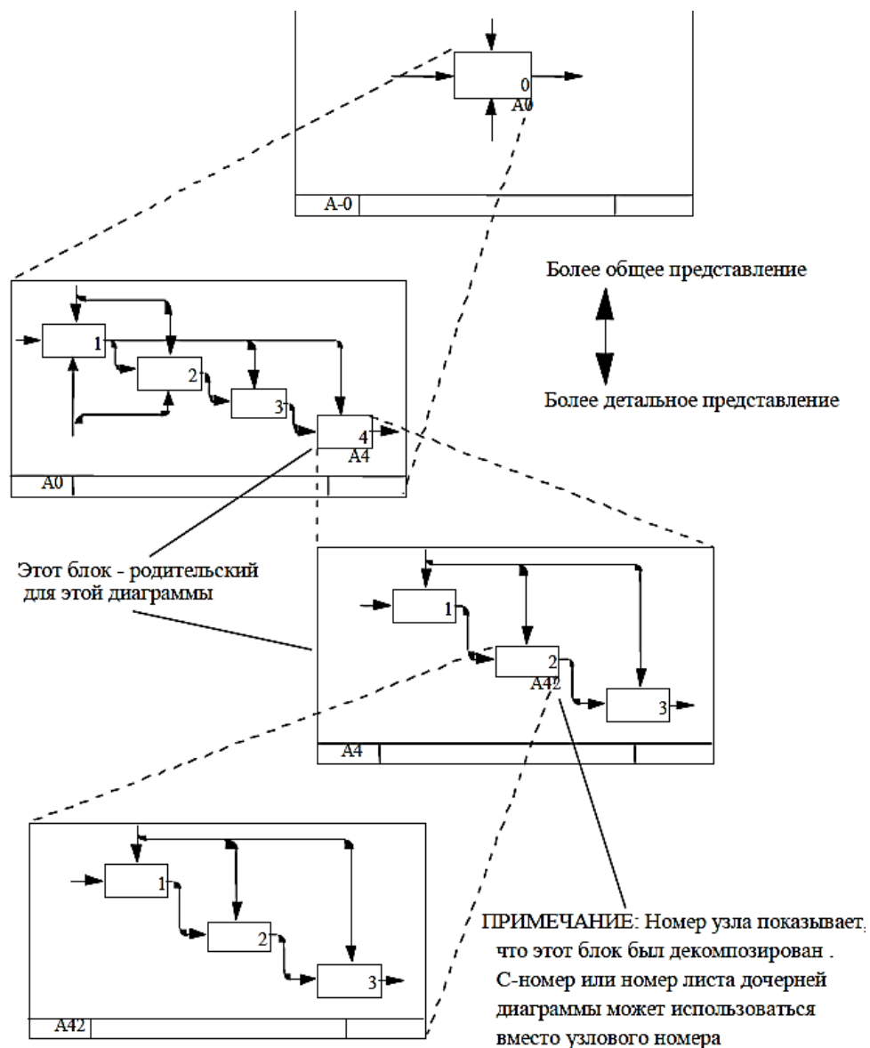
Рис. 4. Операция декомпозиции функциональных блоков в модели IDEF0
